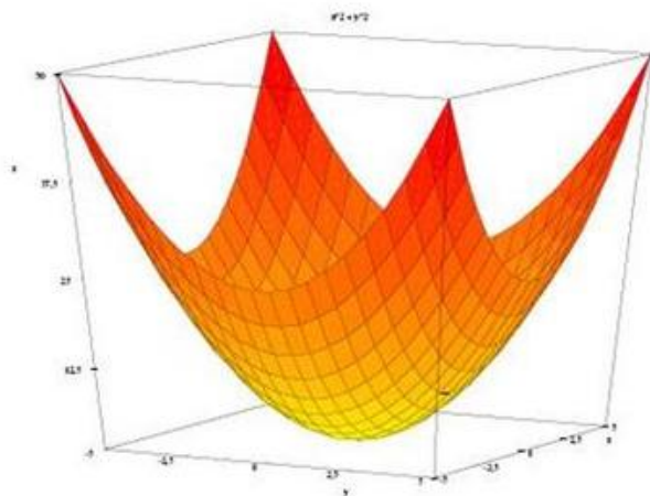
Figura 8: Grafico della funzione f(x, y) = x^2 + y^2
