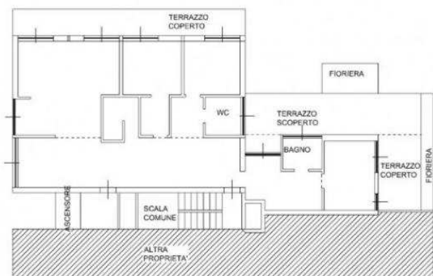
PIANO TERZO SCALA 1:100
