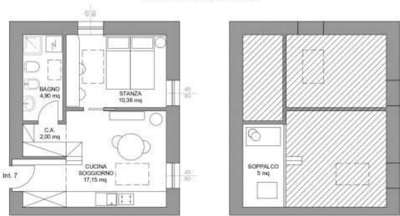
VIA BRENNERO, 28 PIANTA PIANO TERZO
