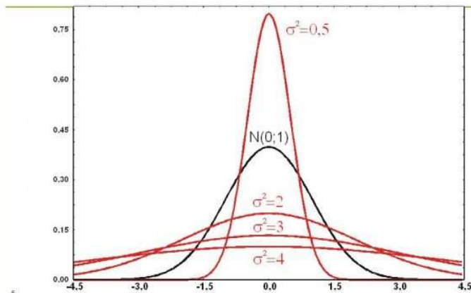
Distribuzione Normale
