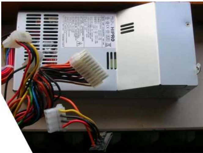
HIPRO HP-U262FF5 REV: X04 AC INPUT(47-63Hz): 100-127V 6A 200-240V 3A MAX. OUTPUT POWER: 260W Perfettamente funzionante
