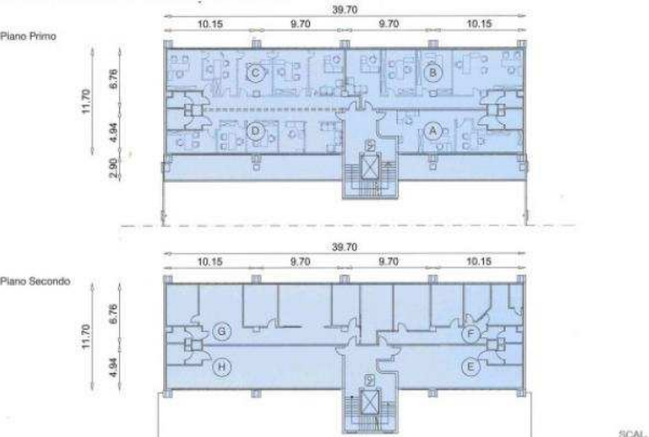
Pianta Piano Primo e Secondo
