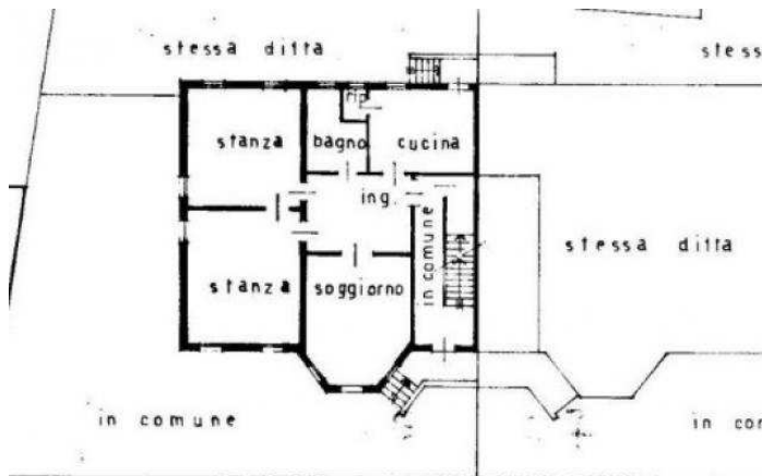
PIANTA PIANO TERRA H=300
